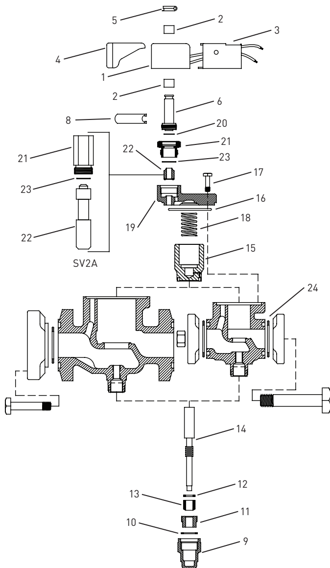
FIG. : SV2 Solenoid Valve
